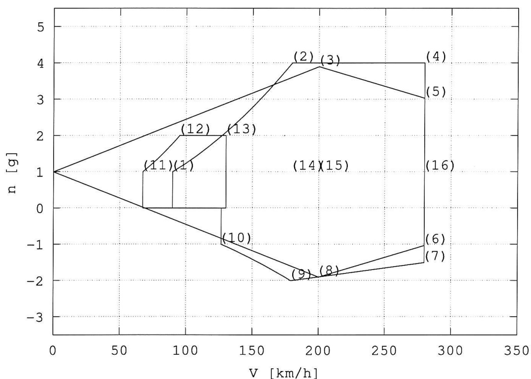
Obrázek: 4. Kombinovaná obálka, m=600,0 kg
